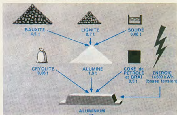
Fabrication de l'aluminium, schéma d'ensemble
