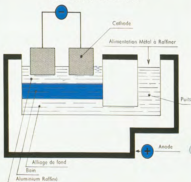
Schéma d'une cuve d'aluminium raffiné
